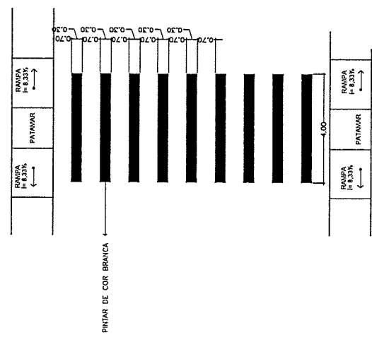
DETALHE DAS FAIXAS DE PEDESTRE SEM ESCALA
